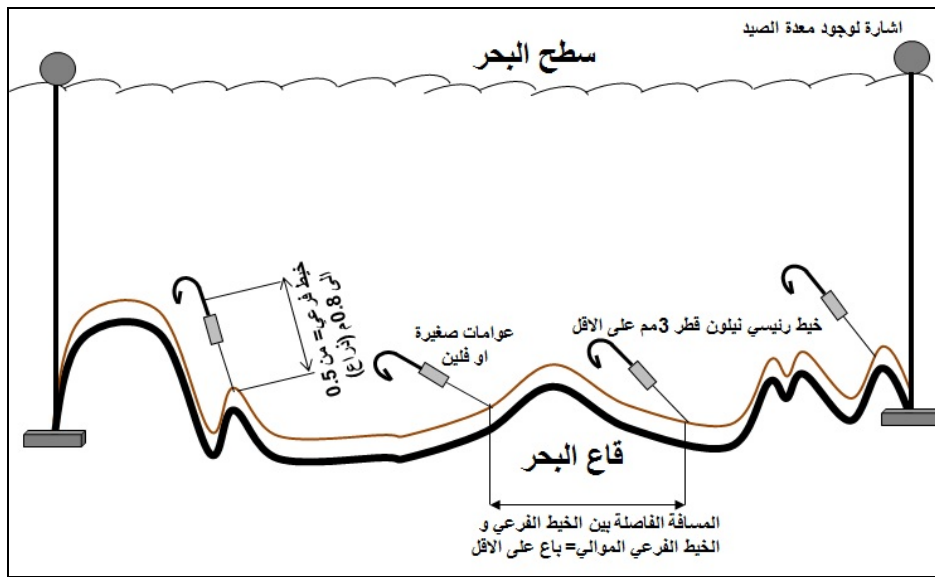
شكل رقم (21): استعمال الخيوط الطويلة على القاع الرملي
