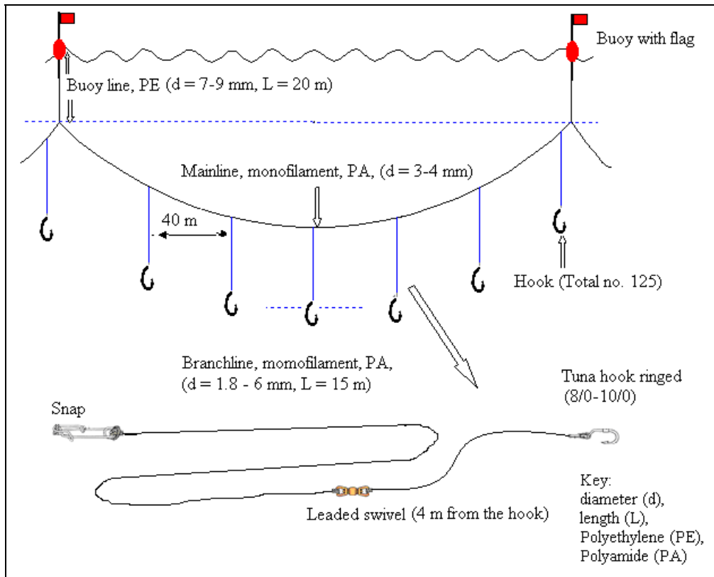
شكل رقم (23): مكونات الخيوط الطويلة السطحية
